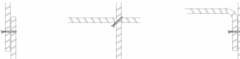
د- اتصال با سیم معمولی ۲۶ (مناسب فقط برای اهداف EMC)
